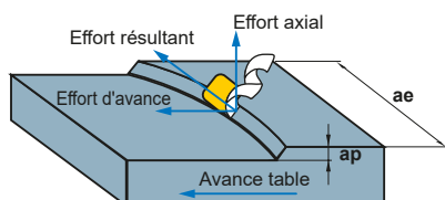
Trois efforts de coupe en présence en fraisage
